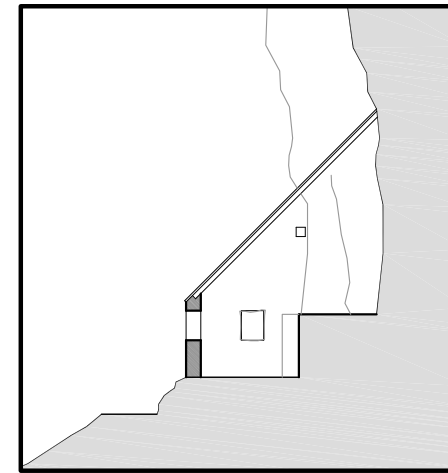
SEZIONE B-B'
