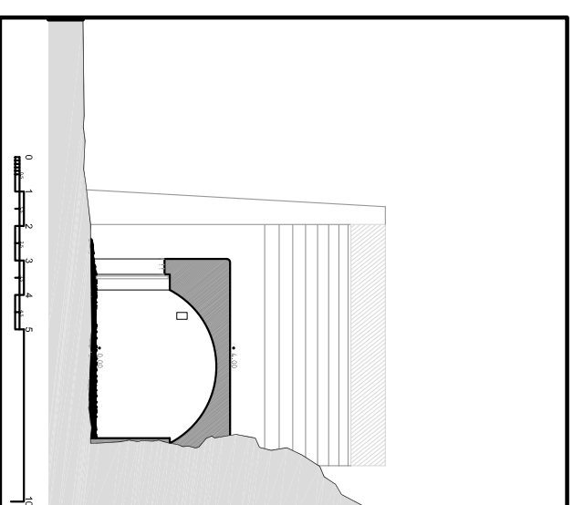
SEZIONE TRASVERSALE
