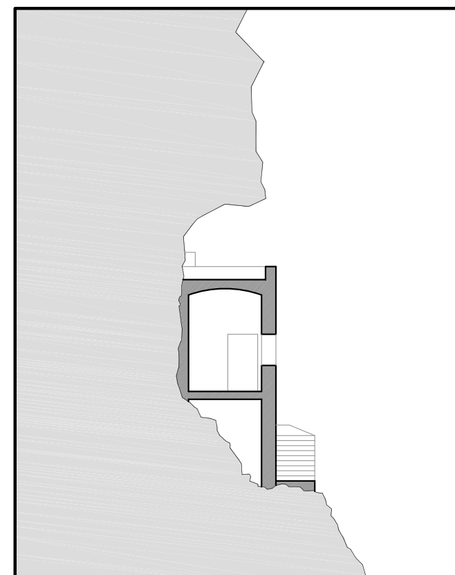
SEZIONE A-A'
