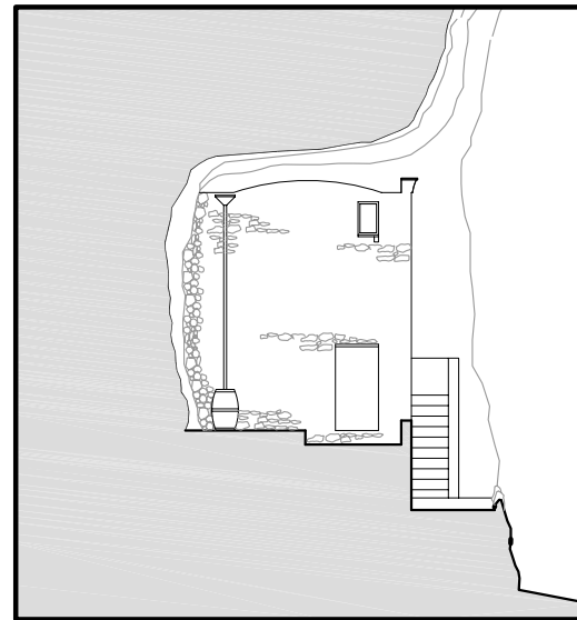
SEZIONE B-B'
