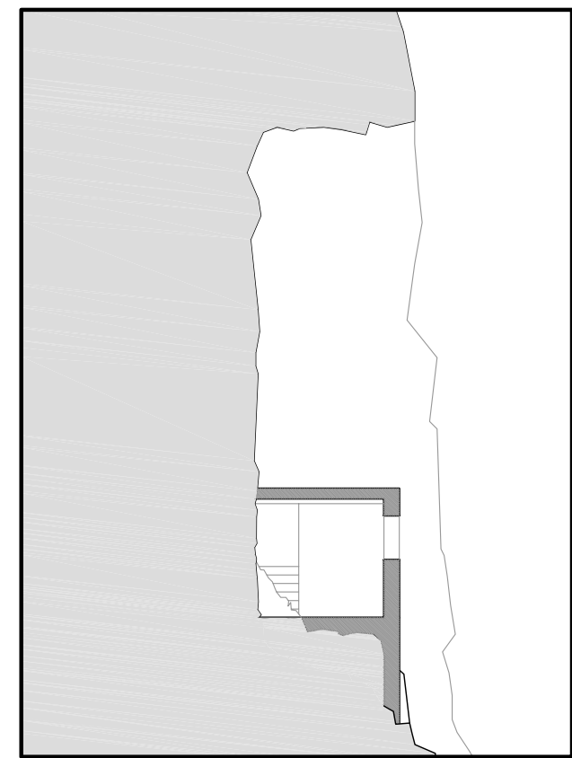
SEZIONE A-A'
