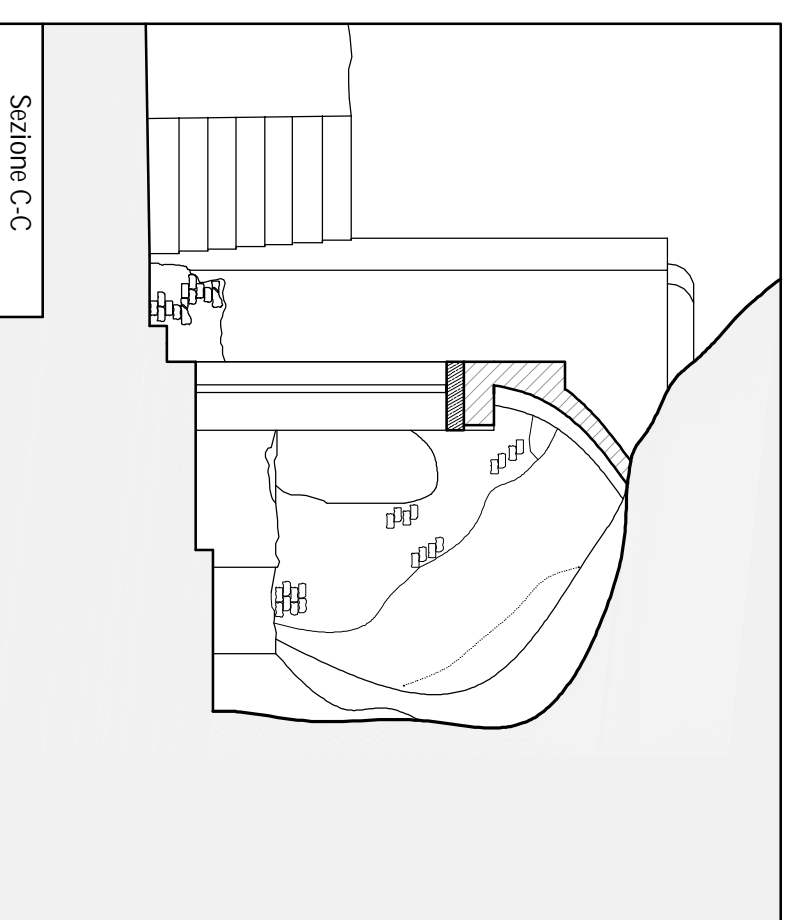
CISTERNA E LAVATOIO A SERVIZIO DELLA CASA
